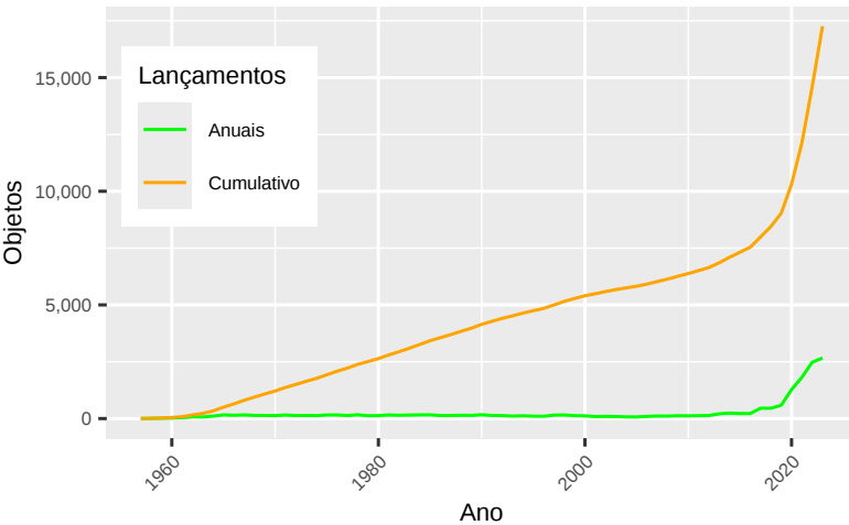
Figura 8.6: Lançamentos anuais e cumulativo de objetos ao espaço, segundo o United Nations Office for Outer Space Affairs (2024).
